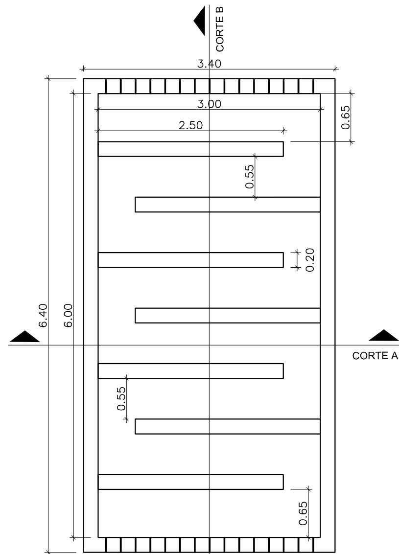
CAIXA DE TRATAMENTO PASSIVO FORMA - PLANTA ESC. 1:50 *PREVER COBERTURA DA CAIXA DE TRATAMENTO PASSIVO DE CHORUME COM TELHAS DE FIBROCIMENTO.
