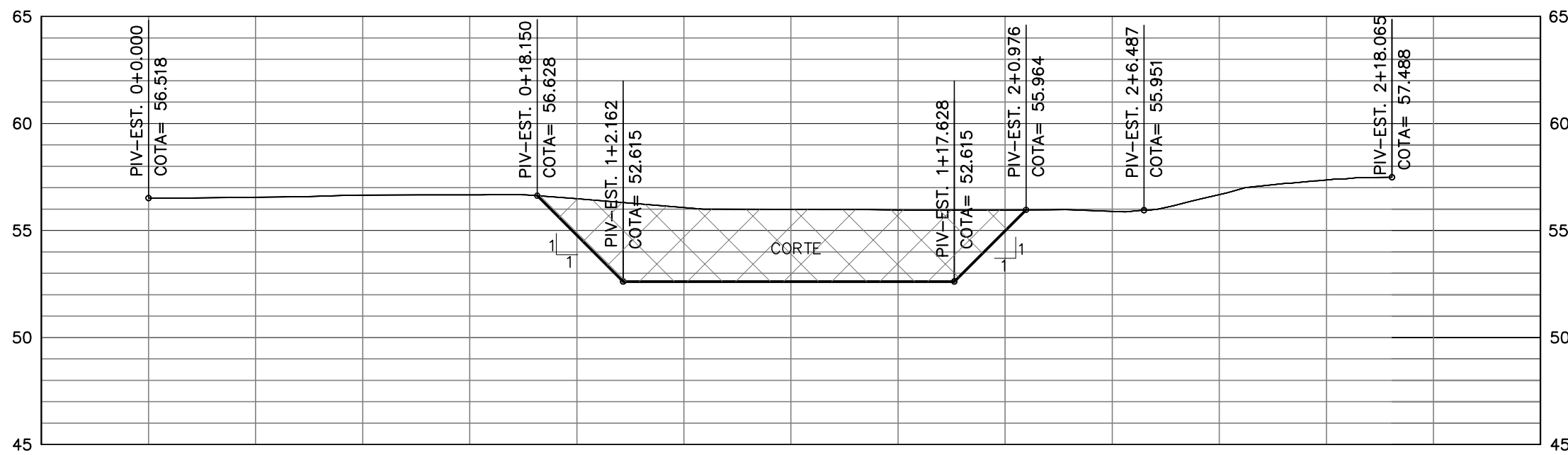
SEÇÃO 3 ESC. H=1:250
