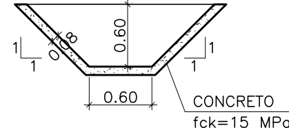
CANALETA DR-3B-13 SEM ESCALA (VER NOTA 16)
