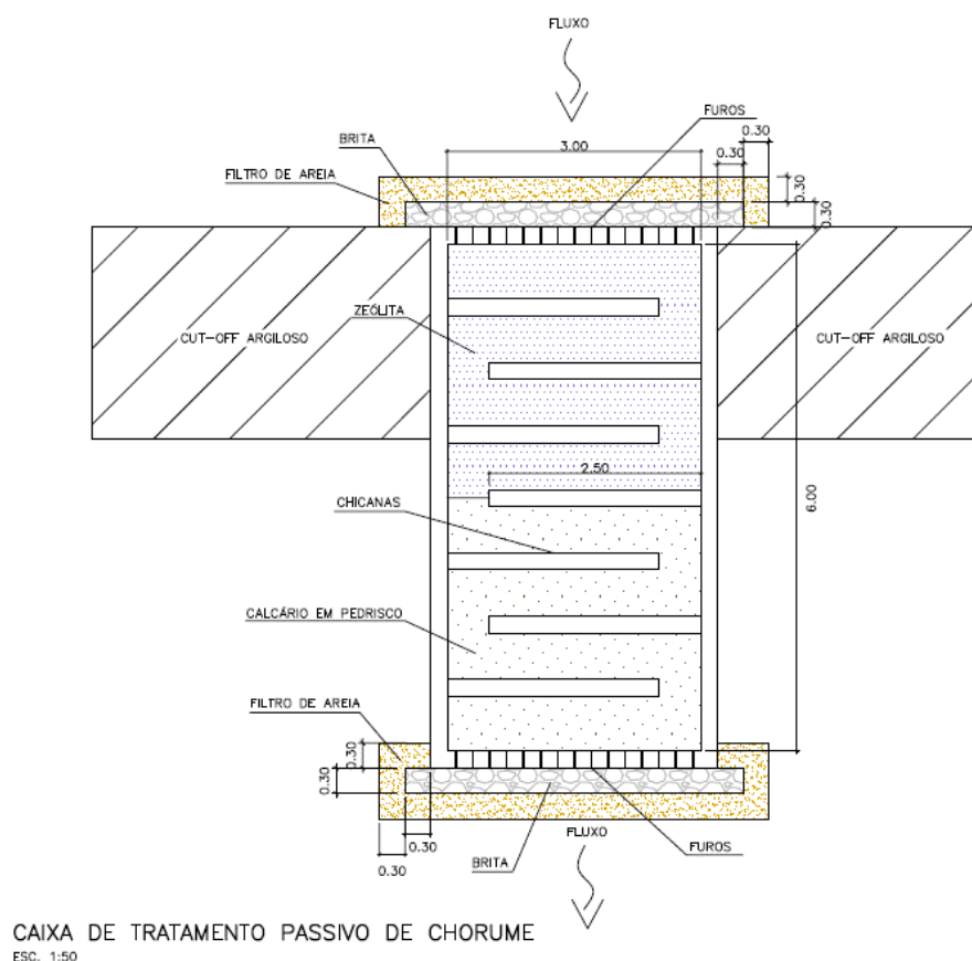
Figura 5.4 – Vista do tanque de tratamento passivo.
