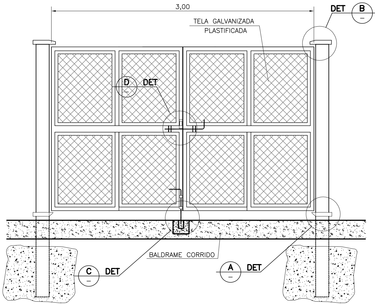
DETALHE GENÉRICO DO PORTÃO ESC.: SEM ESCALA
