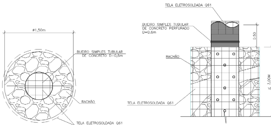
Figura 5.5 - Detalhe dos drenos de gás.
