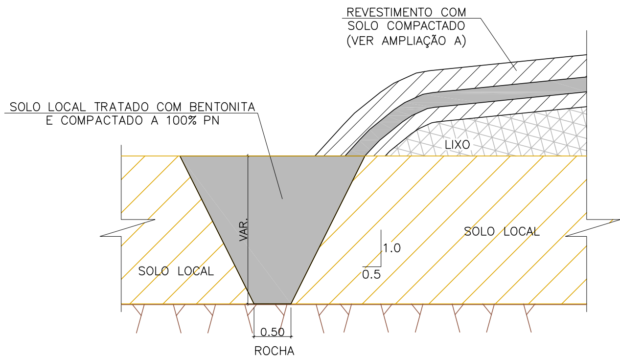
DETALHE DO CUTOFF ARGILOSO PARA ENCAPSULAMENTO SEM ESCALA (VER NOTA 16)
