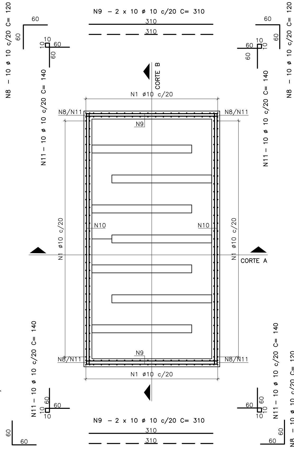
CAIXA DE TRATAMENTO PASSIVO DE CHORUME ARMAÇÃO - PLANTA ESC. 1:50
