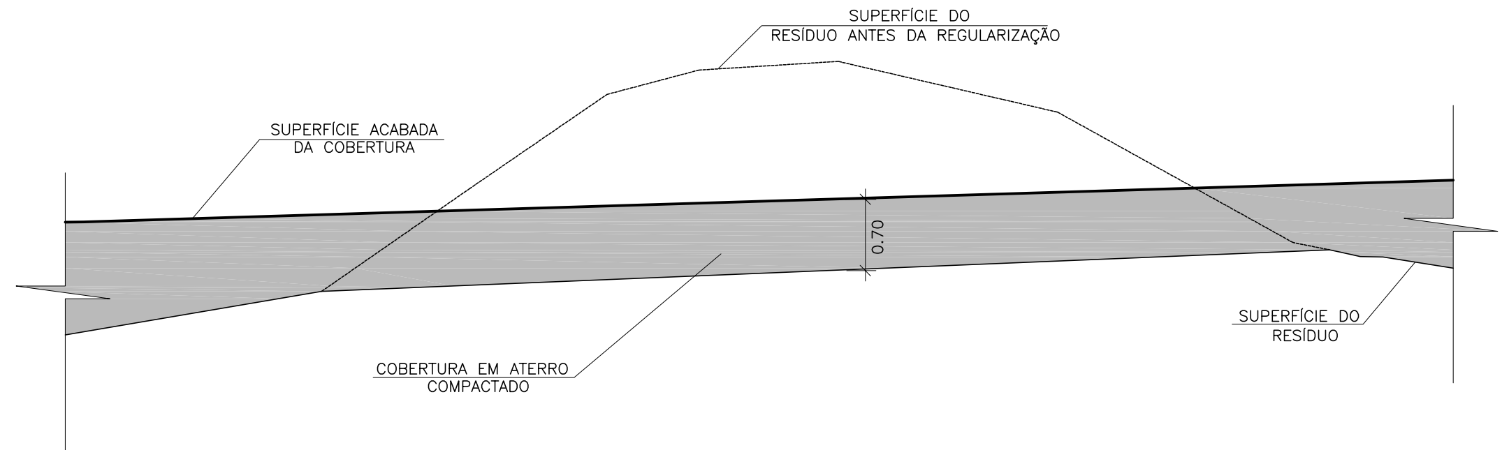
DETALHE DE TRATAMENTO NAS REGIÕES DE CORTE SEM ESCALA (VER NOTA 19 E 20)
