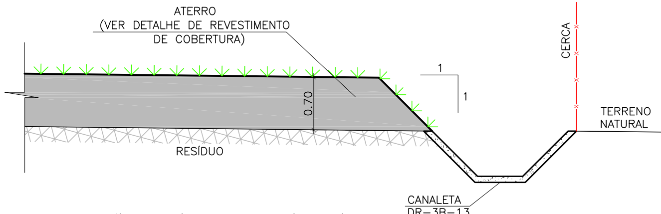
AMPLIAÇÃO A (DETALHE TÍPICO) ESC. 1:50
