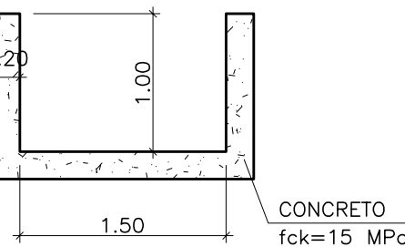
CANAL DE ESCOAMENTO RETANGULAR TIPO R2.1 SEM ESCALA (VER NOTA 16)
