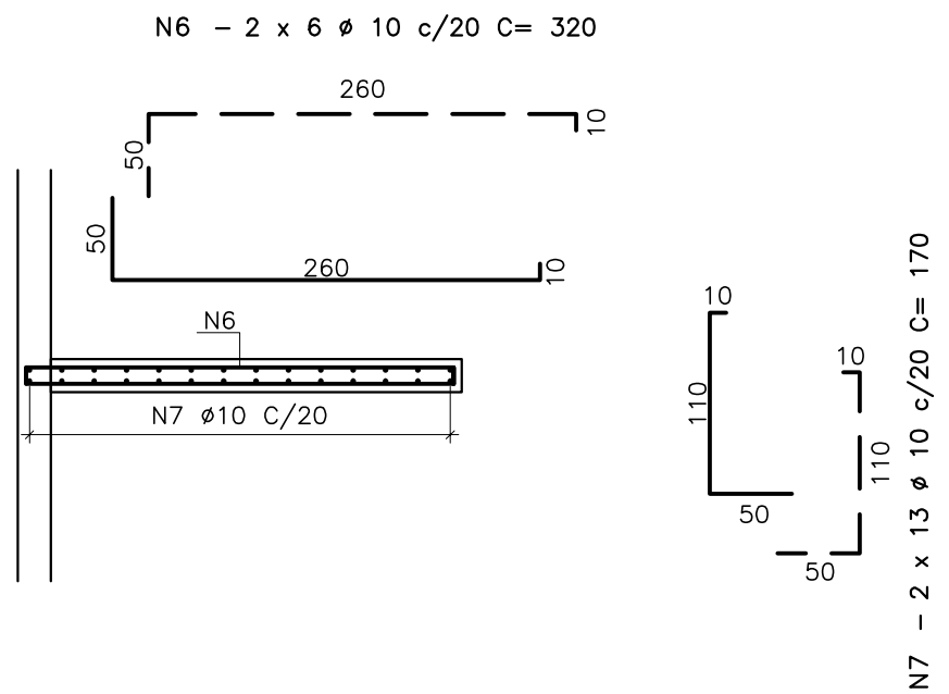
CAIXA DE TRATAMENTO PASSIVO DE CHORUME ARMAÇÃO CHINACAS (x7) ESC. 1:50
