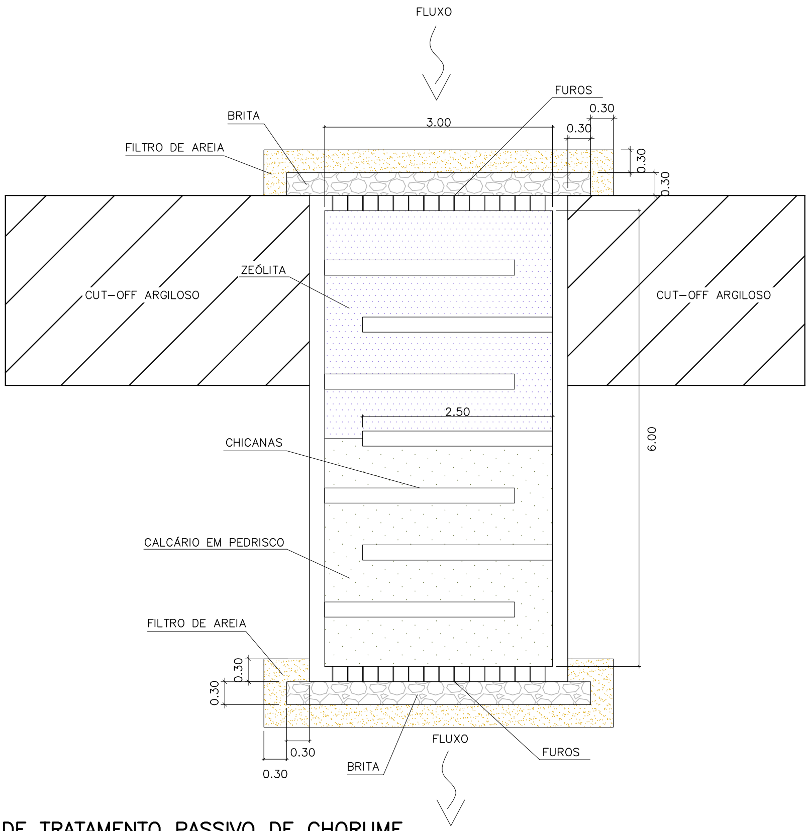
CAIXA DE TRATAMENTO PASSIVO DE CHORUME ESC. 1:50 *PREVER COBERTURA DA CAIXA DE TRATAMENTO PASSIVO DE CHORUME COM TELHAS DE FIBROCIMENTO.
