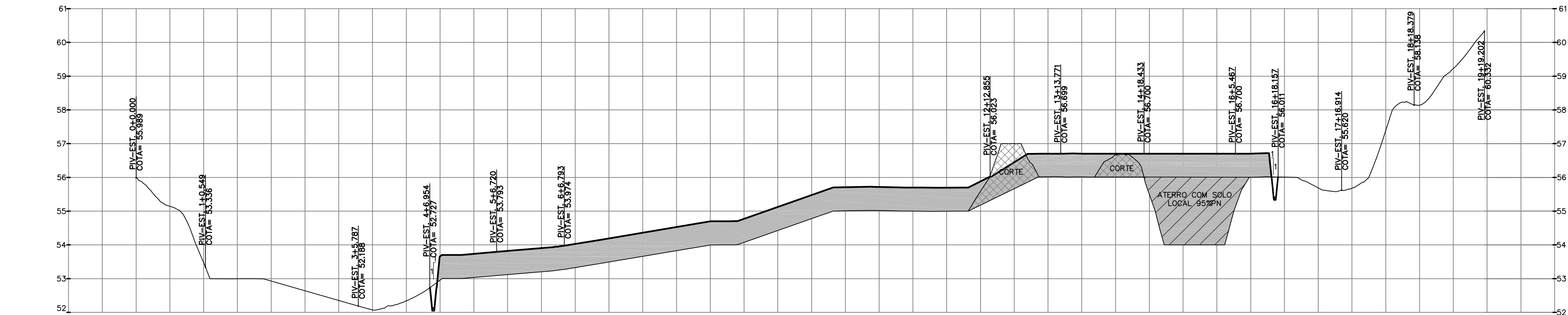
SEÇÃO 2 ESC. H=1:1000/V=1:100
